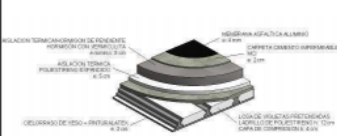
1 Detalle Techo
